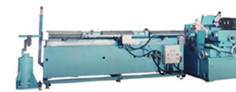
8 長棒研磨裝置
