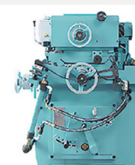
11 停止式研磨自動進退刀裝置
